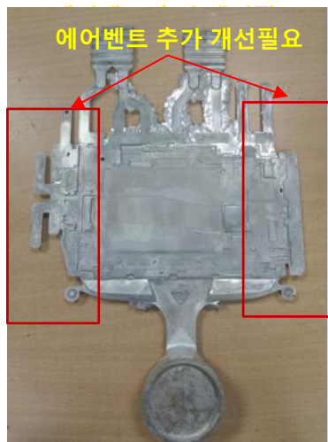
캐스팅 상태 (전면)
