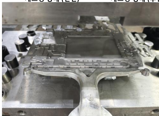
디게이팅 트리밍에 제품 안착 후 모습
